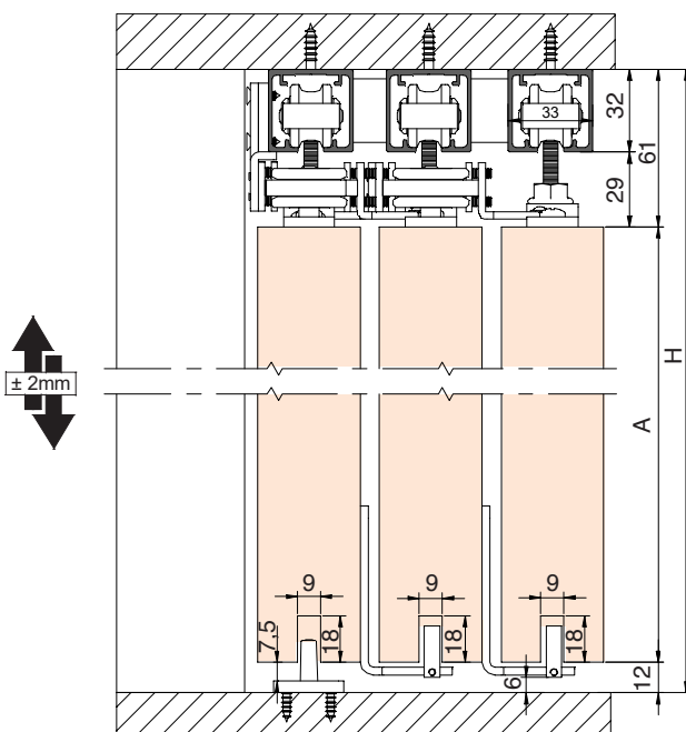
SF-TELESCÓPICA PROGRESIVA 3 HOJAS | PANELS | PANNEAUX
