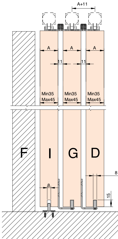
SF-TELESCÓPICA 3 HOJAS I PANELS I PANNEAUX
