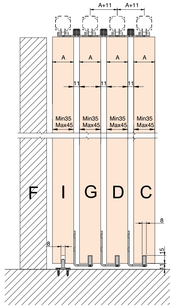
SF-TELESCÓPICA 4 HOJAS I PANELS I PANNEAUX
