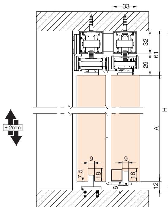
SF-TELESCÓPICA PROGRESIVA SINCRO 2+2 HOJAS | PANELS | PANNEAUX
