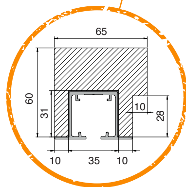
SECCIÓN PERFIL STAR FT ENCASTRADO EN MADERA
