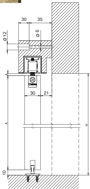
SECCIÓN PERFIL STAR FT ENCASTRADO EN MADERA
