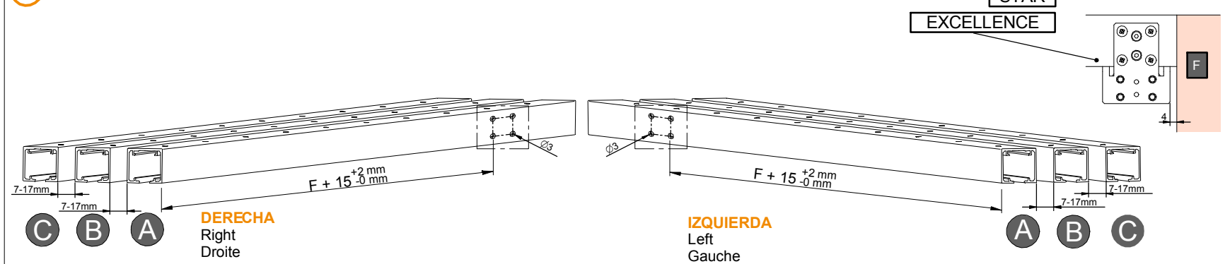
1 MONTAJE PERFILERIA / Profile assembly / Assemblage profil
