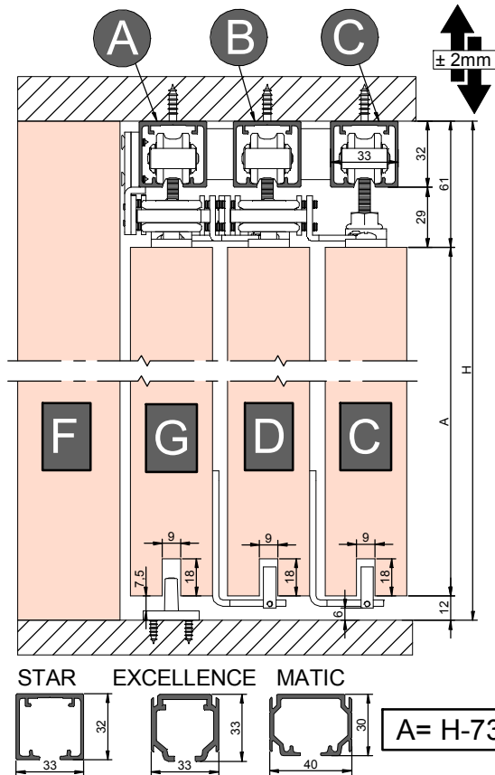
2 MONTAJE PERFILERIA / Profile assembly / Assemblage profil
