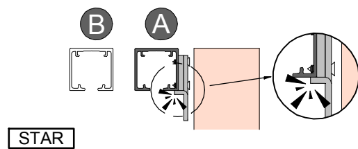
2 MONTAJE PERFILERIA / Profile assembly / Assemblage profil
