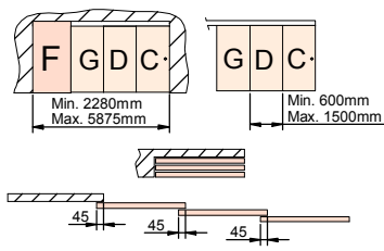
ENRASADO / Leveled / Arasé
